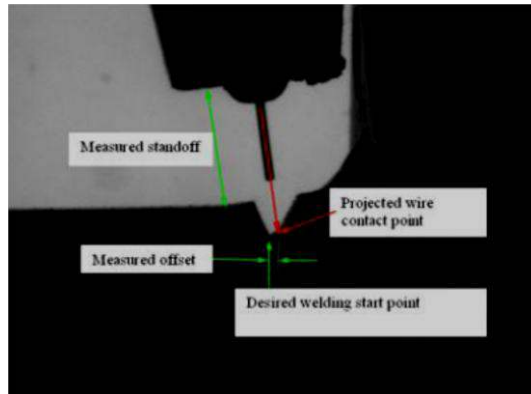
Fig.2 Welding parameters
