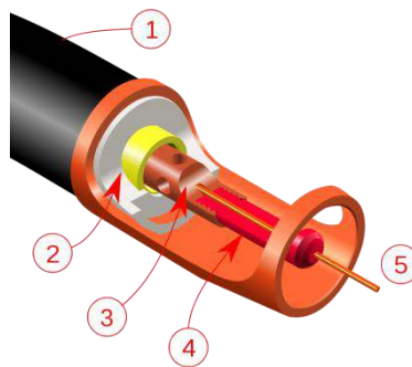
Fig. 3 GMAW torch
