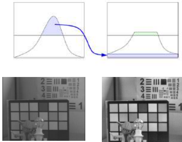
Fig.21 CLAHE
